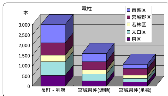
図-5-12 通信施設の被害量（電柱、および架空ケーブル）
