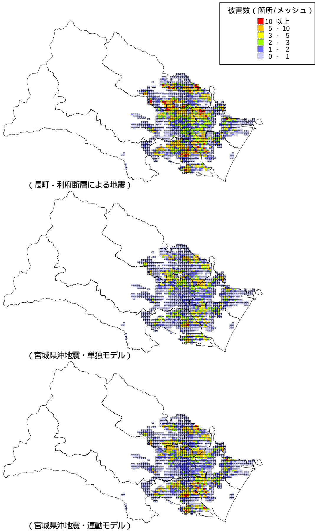
図 - 5 - 7 ガス導管（低圧導管）の被害分布
