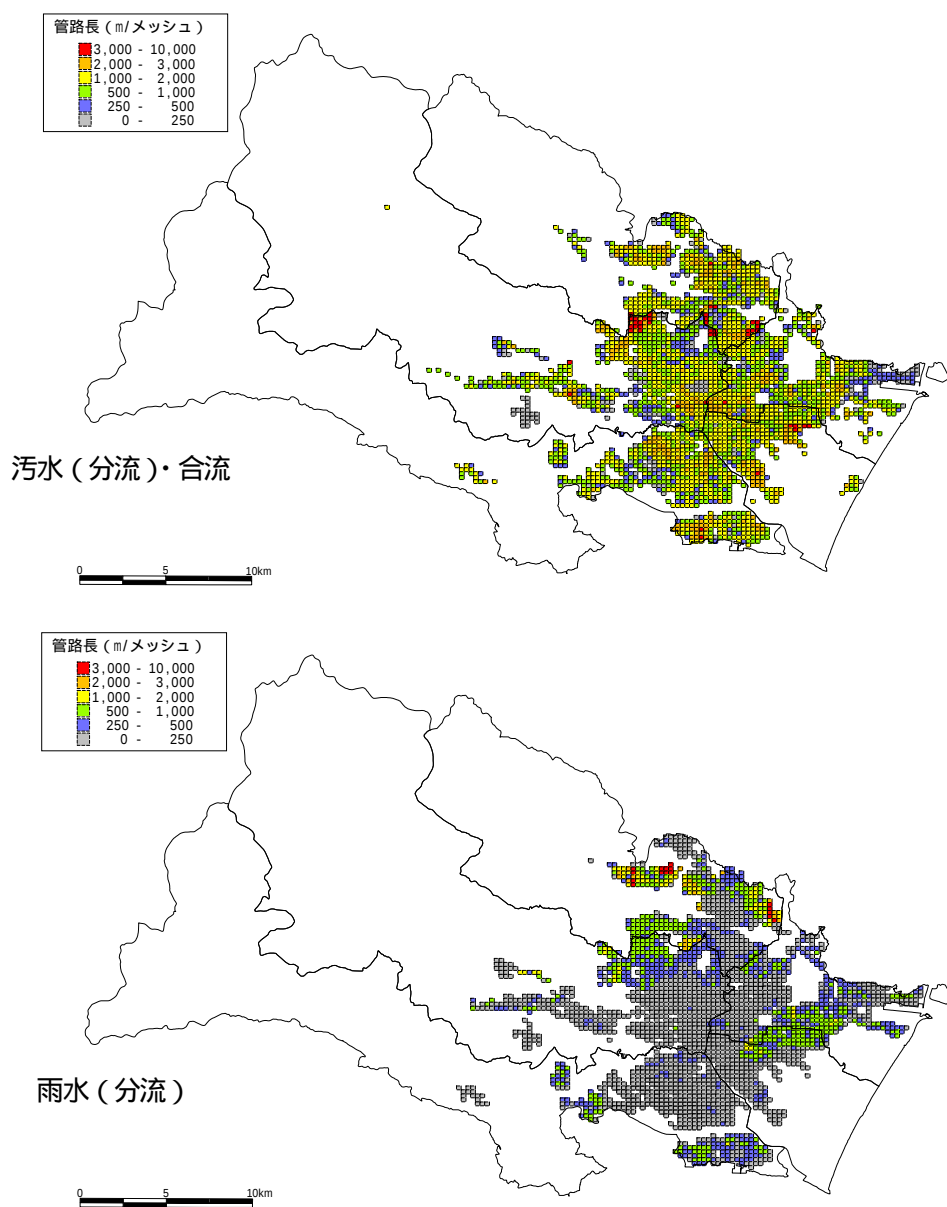
図 - 5 - 3 下水道 (汚水 (分流)・雨水 (分流)) の延長分布図
