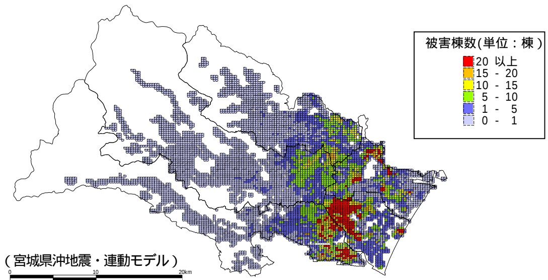
図 - 1 - 5 木造建物の半壊・中破棟数分布
