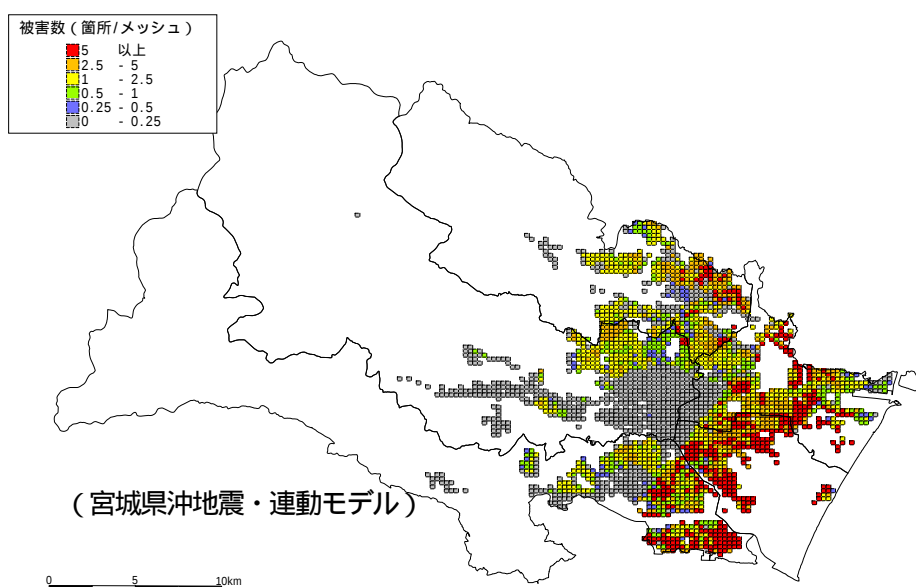
図 - 5 - 4 下水道管 (汚水 (分流)・合流) 被害分布
