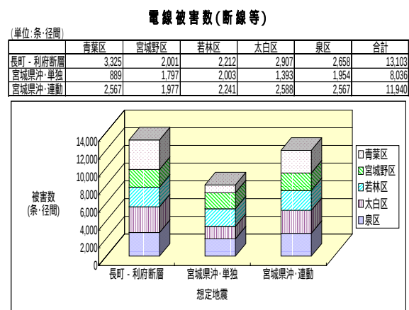
図 - 5 - 10 電線設備被害(架空)
