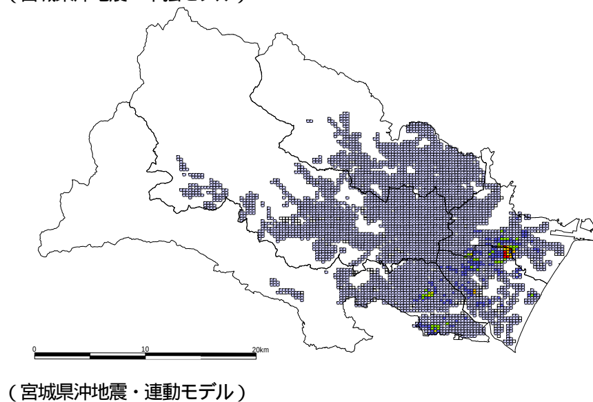
図 - 5 - 2 上水道（送・配水管）被害分布
