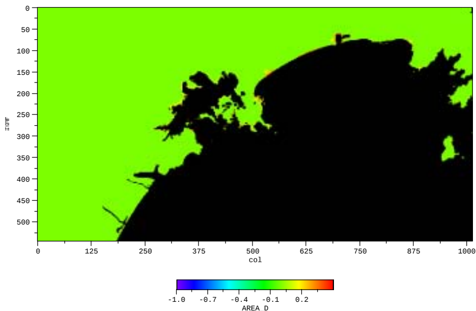
図 - 2(a) 津波遡上分布図（単独モデル）
