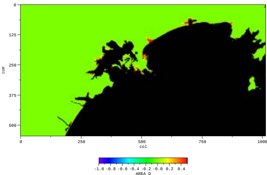
図 - 2(b) 津波遡上分布図（連動モデル）
